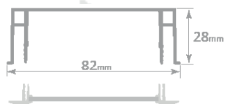
Профіль парящі лінії 90мм з оргсклом та вставкою 2.0
