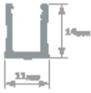
Штапиковий профіль 2.5
